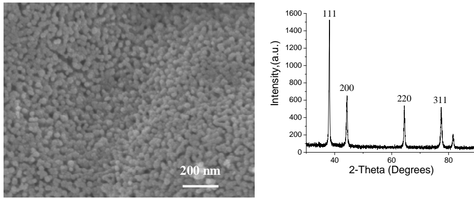
图 S1 Ag 纳米管的 SEM 图像和 XRD 谱图 Fig.S1 SEM image and XRD spectrum of Ag nanotubes
