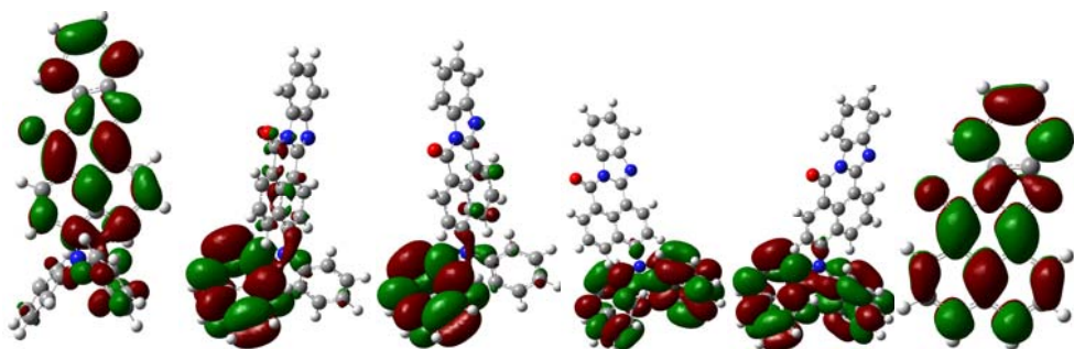
VI-LUMO+1 VII-LUMO+1 VIII-LUMO+1 IX-LUMO+1 X-LUMO+1 XI-LUMO+1
