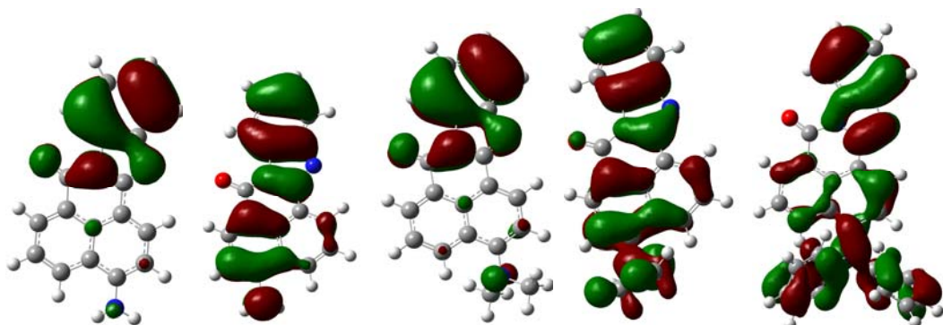
I-HOMO-1 II-HOMO-1 III-HOMO-1 IV-HOMO-1 V-HOMO-1
