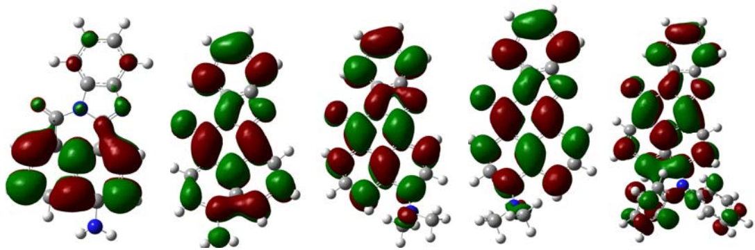
I-LUMO+1 II-LUMO+1 III-LUMO+1 IV-LUMO+1 V-LUMO+1
