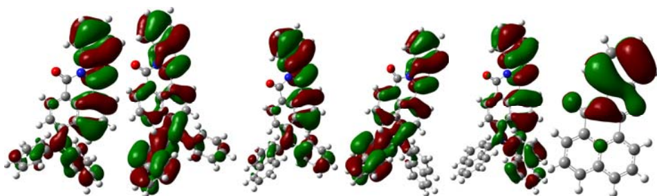
VI-HOMO-1 VII-HOMO-1 VIII-HOMO-1 IX-HOMO-1 X-HOMO-1 XI-HOMO-1
