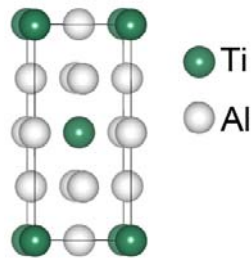
图 S2 \text{Al}_3\text{Ti} 的晶体结构图
