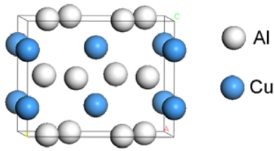
图 S1 \text{Al}_2\text{Cu} 的晶体结构图
