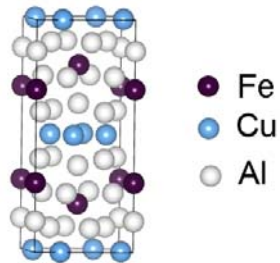
图 S3 \text{Al}_7\text{Cu}_2\text{Fe} 的晶体结构图
