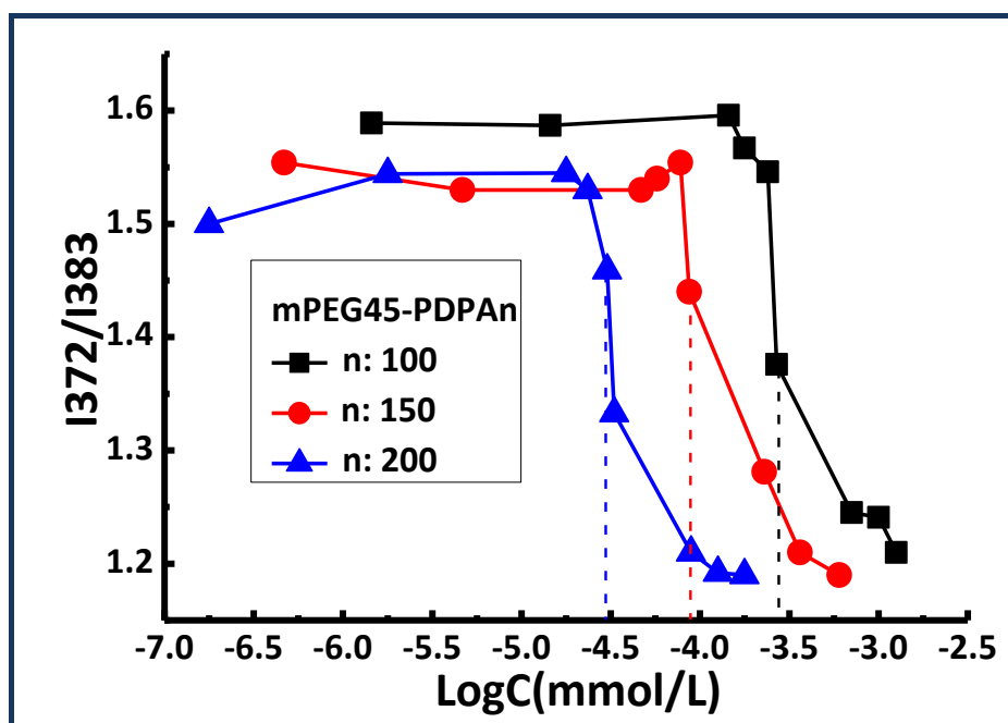
图S1 不同嵌段聚合物的临界胶束浓度 (CMC)
