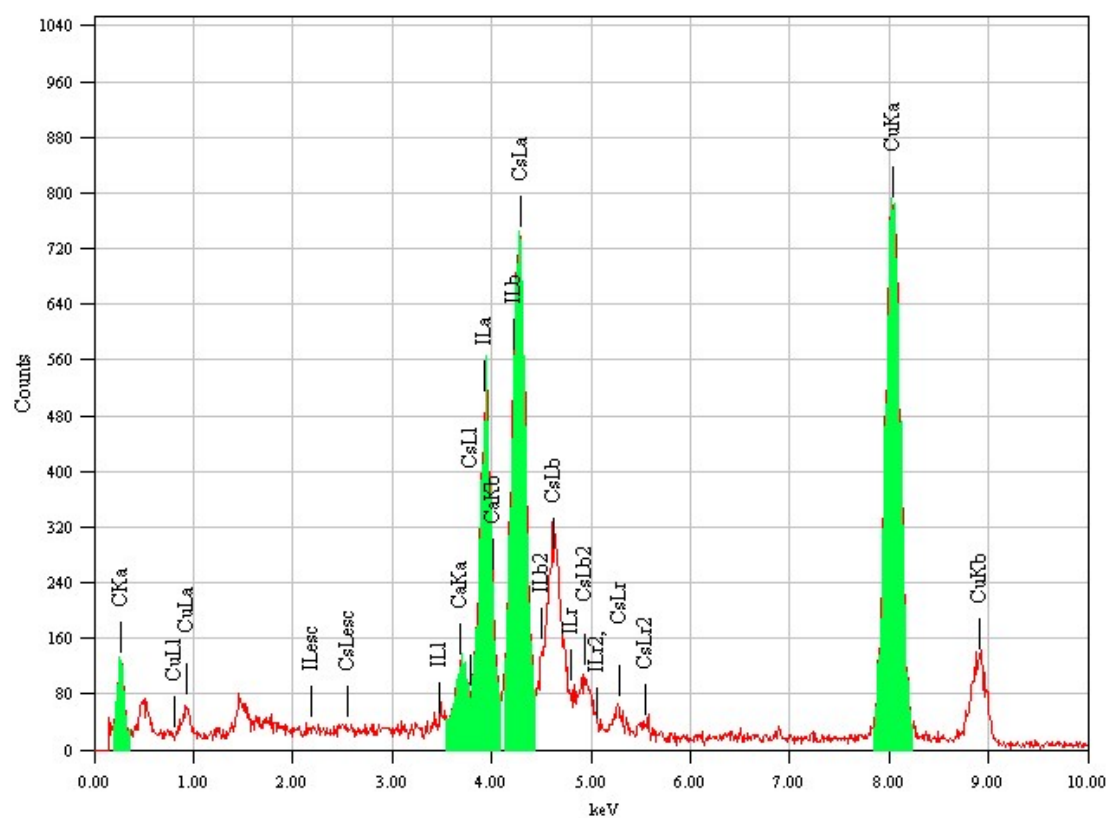
该图为样品 TEM 图像对应 CsI 区域内的 EDS 结果，此结果证实了 TEM 图像中 CsI 的存在。
